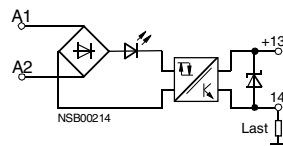
3TX7 00.-3AB04
