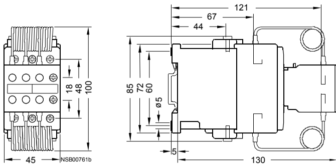
Fig. 3-93: 3RT16 27
