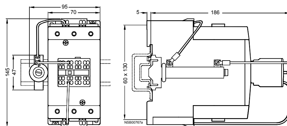
Fig. 3-98: 3RT10 4
