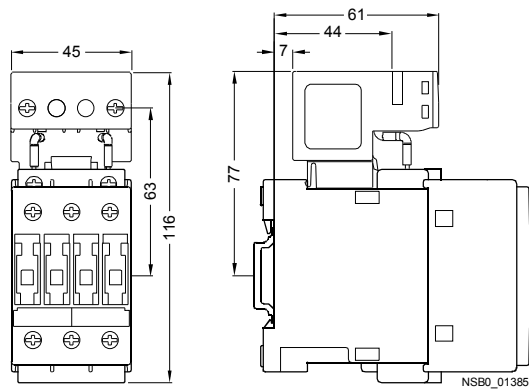
Fig. 3-100: 3RT10 2.-1X.40-0LA2
