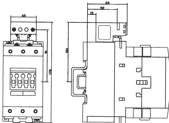
Fig. 3-104: 3RT10 4.-1X.40-0LA2
