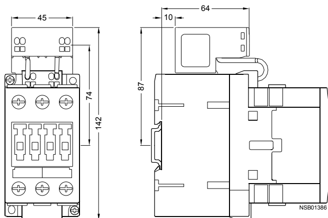
Fig. 3-101: 3RT10 3.-3X.40-0LA2
