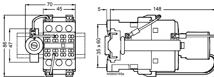
Fig. 3-96: 3RT10 2
