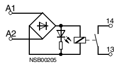
3TX7 00.-1M.00
