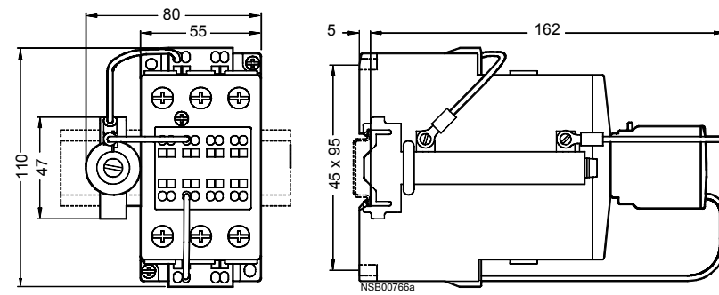
Fig. 3-97: 3RT10 3
