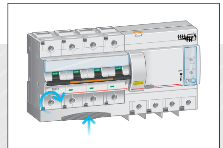
ЗАТЯНИТЕ ЗАЖИМЫ и установите крышку выводов
